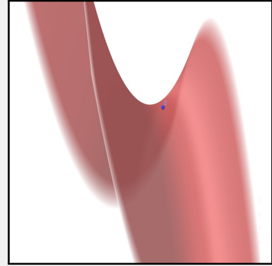
Figura 3.6: Punto silla en z = x^2 - y^2
